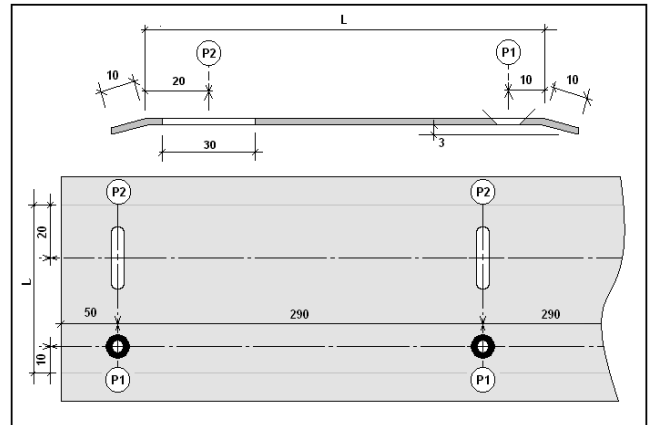
Modèle avec double perçage // Double drilling type
