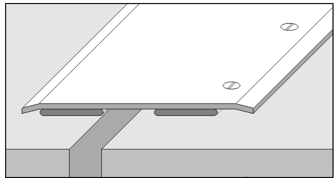
Modèle à perçage unique // Single drilling type avec mastic élastomère pour trafic voitures légères
