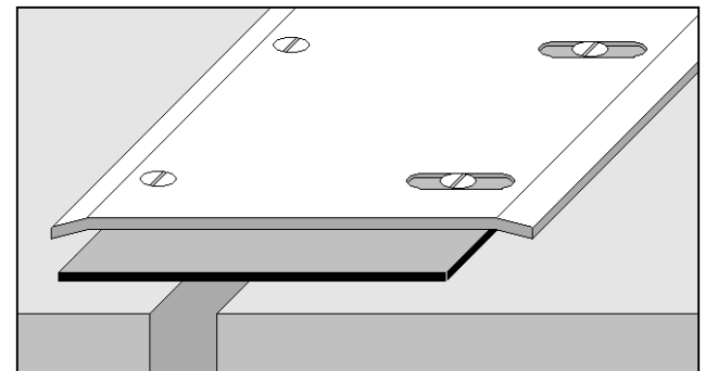
Modèle avec double perçage // Double drilling type avec bande anti-affaissement pour trafic d'engins
