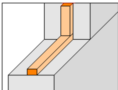
Reprises de bétonnage // Construction joints
